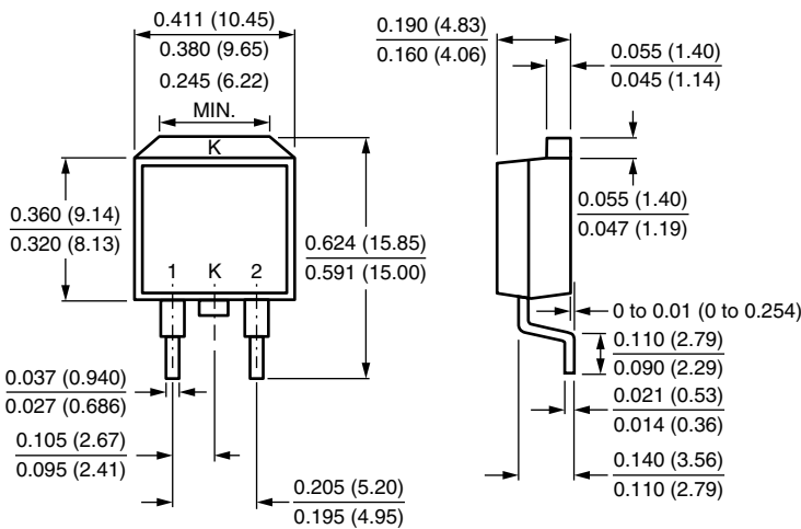
TO-263AB
